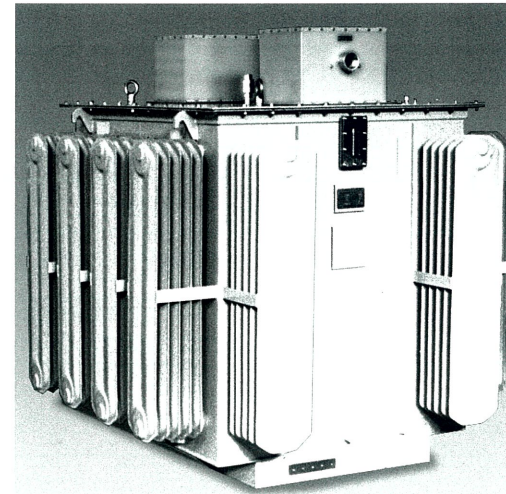
①NCT-G型 200kVA 油浸式
