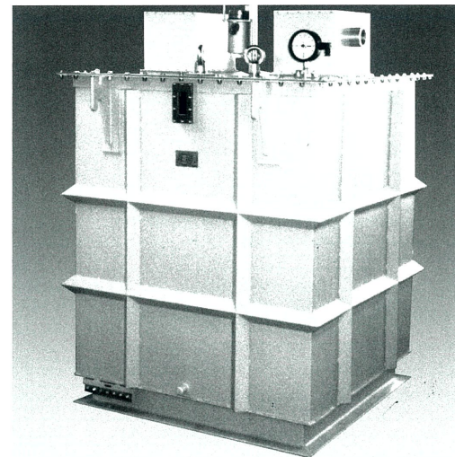
③NCT-F型 短時間1500kVA 油浸式
