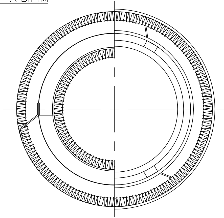
A-A'断面図
