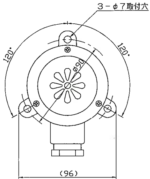
正面図
