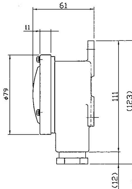
側面図
